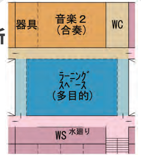
ラーニングスペース（多目的） 3階平面図
