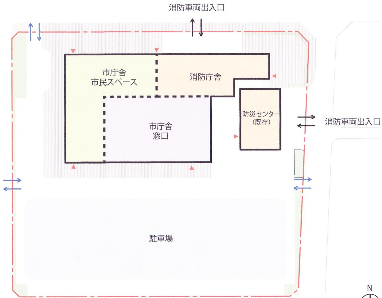
敷地計画概図
