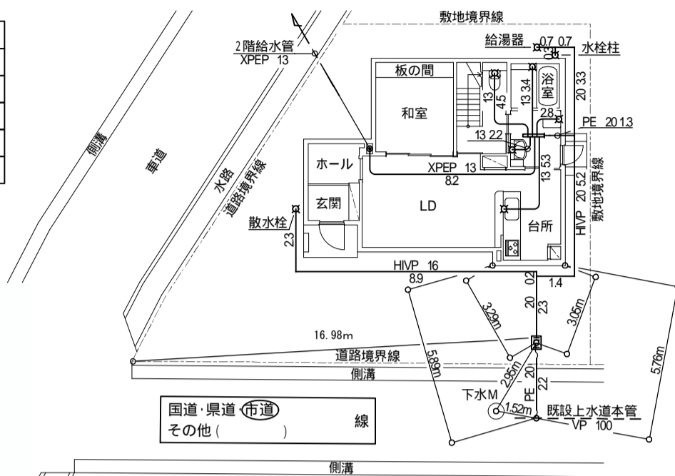
平面図 S=1:200
