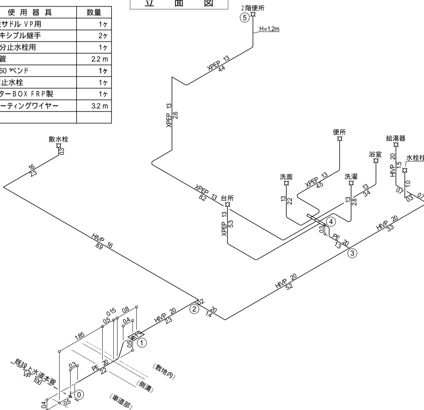
立面図
