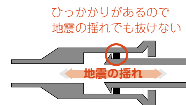
耐震継手の断面図
