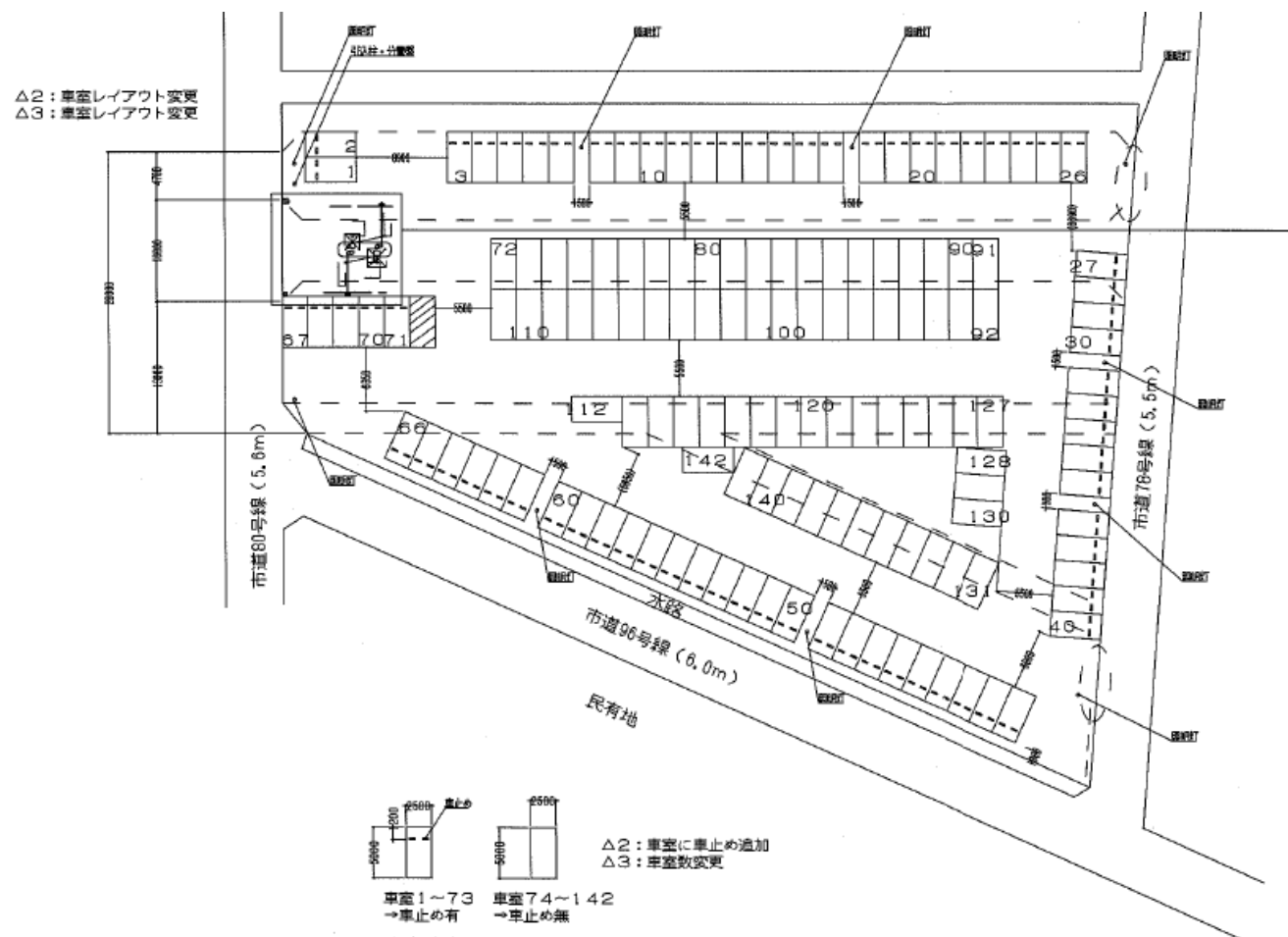
白銀駐車場 平面図
