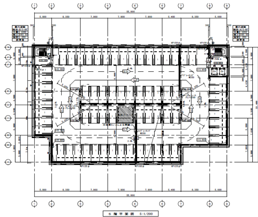
立体駐車場平面図（5階、R階）
