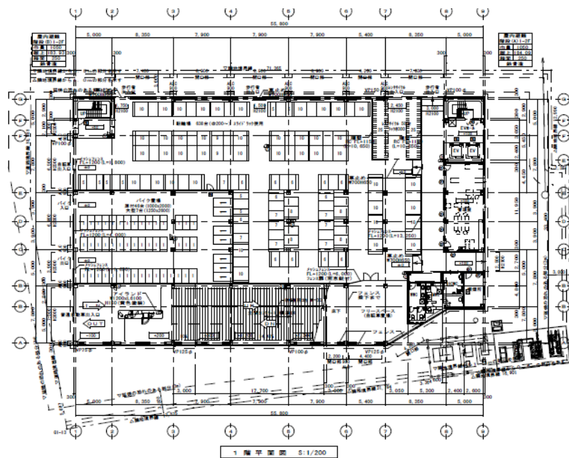
立体駐車場平面図（1階、2階）
