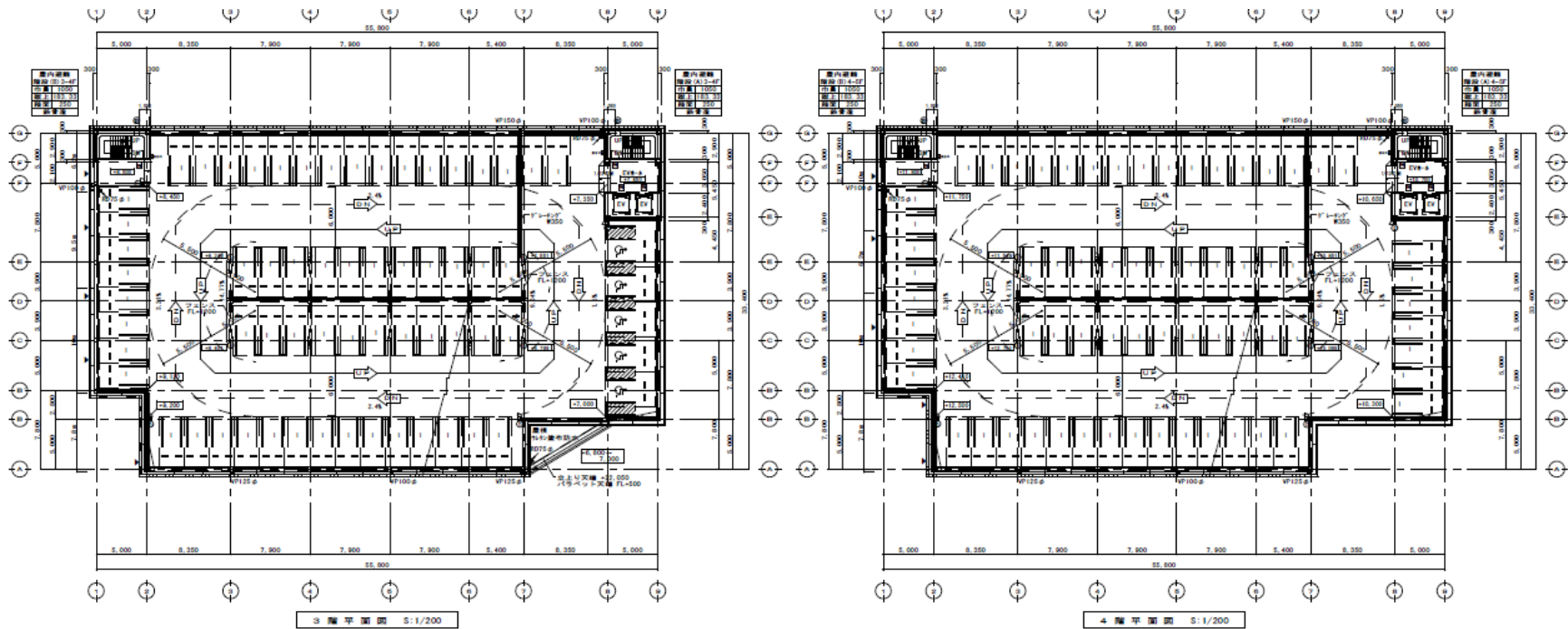
立体駐車場平面図（3階、4階）
