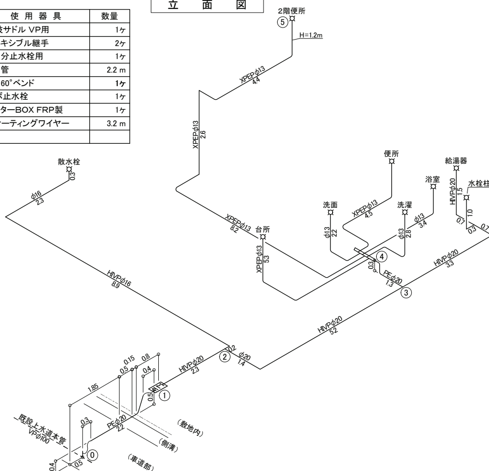
立 面 图
