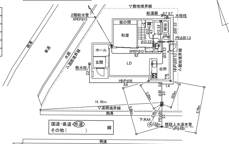
平面图 S=1:200
